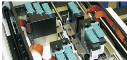
Druckkopfaufteilung
